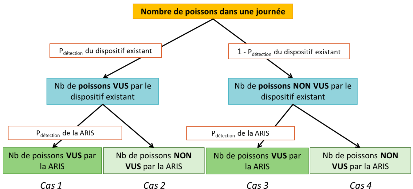
Figure 1 : Structure générale du modèle avec les 4 cas pouvant être observés dans le cadre de l'utilisation de deux dispositifs de comptage
