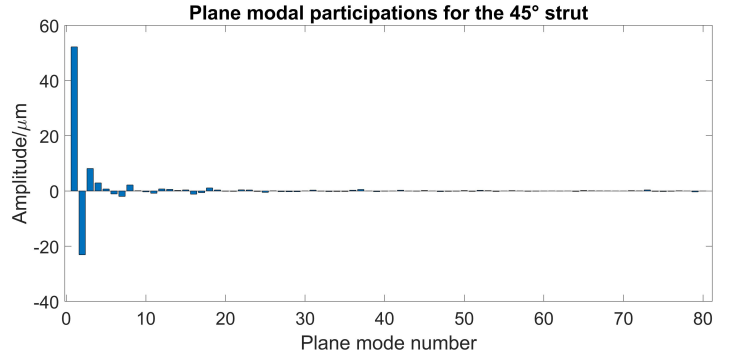
(b) 45° strut
