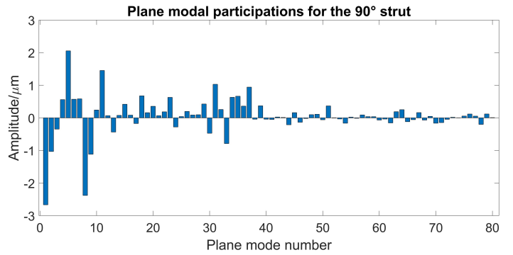
(a) 90° strut
