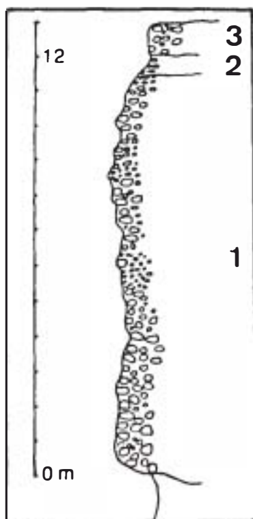
Fig. 2. La terrasse du Pléistocène moyen (bassin de Ksabi): (1) conglomérat de base; (2) cailloutis sans accumulation de carbonate; (3) niveau supérieur induré.
