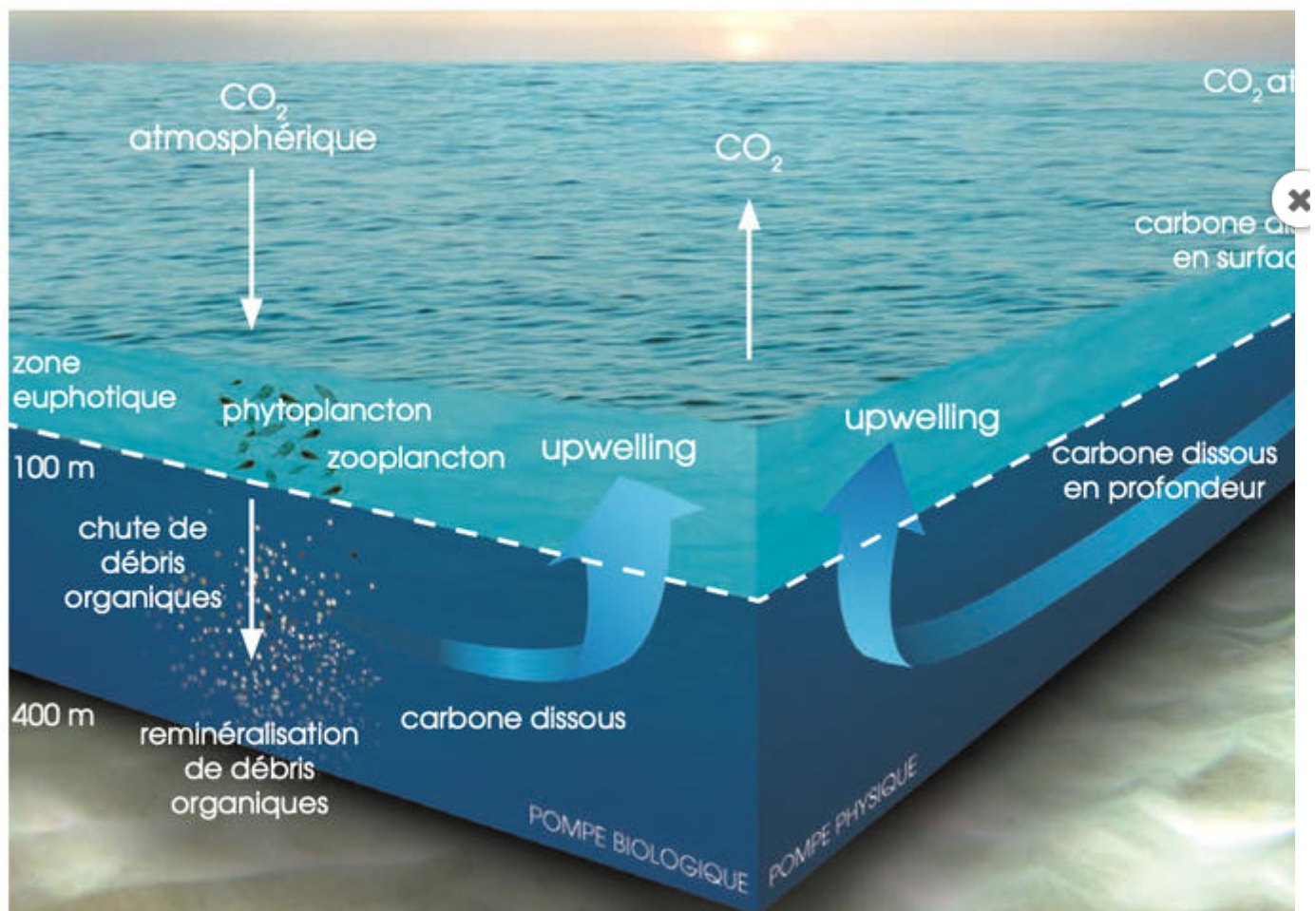
Cycle du carbone naturel et représentation des pompes biologique et physique (Bopp et al. 2002).
