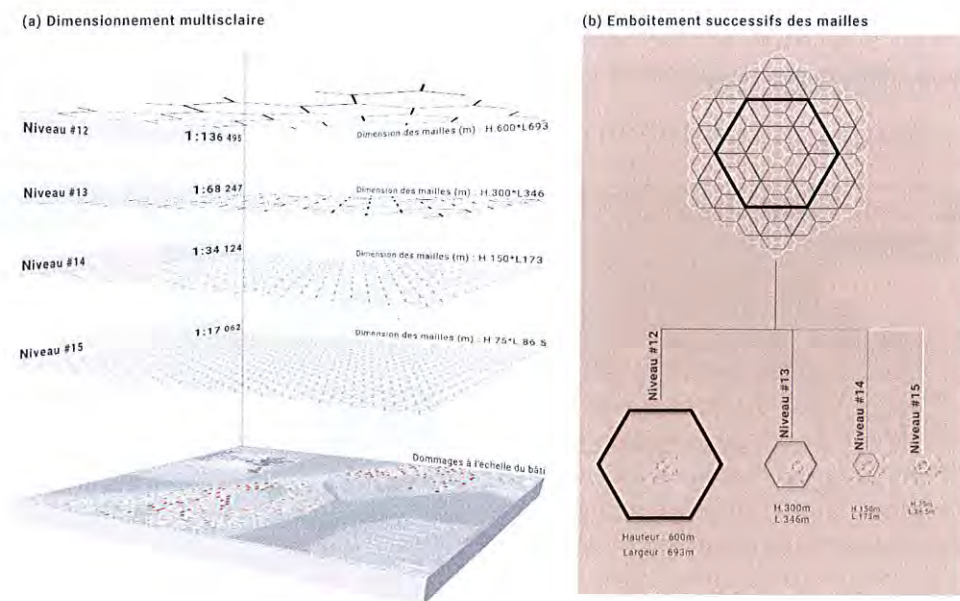
Figure 6 : Schéma de principe du dimensionnement multiscalaire (a) et de l'emboîtement successifs des mailles (b)
