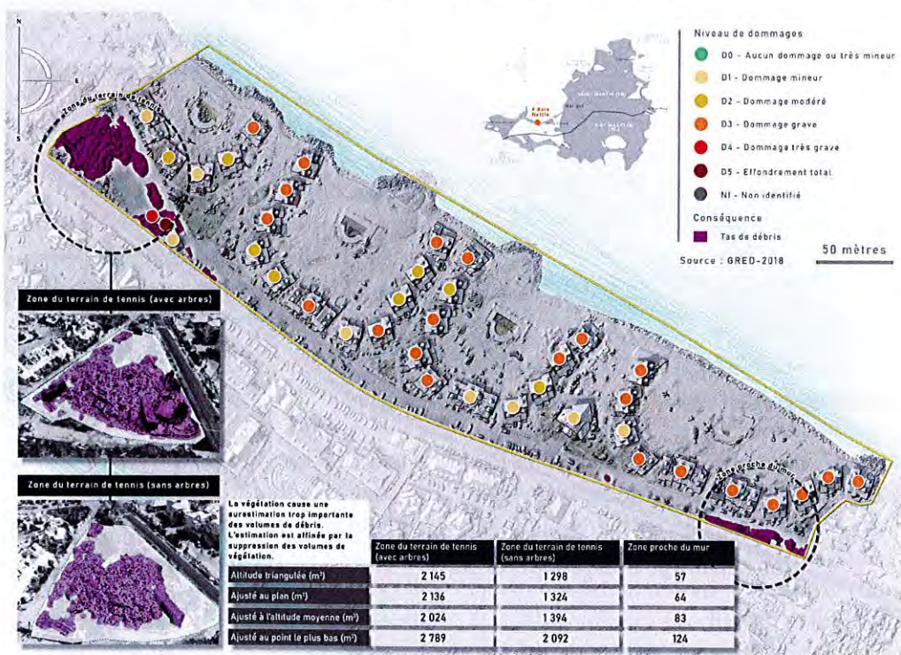
Figure 6 : Exemples de cubage de débris cycloniques à partir de traitements photogrammétriques d'images acquises par drone (Saint-Martin)
