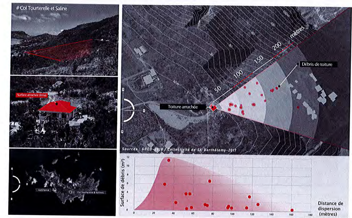
Figure 3 : Analyse de la dispersion de débris de toitures au moyen d'un drone (Saint-Barthélemy)
