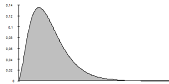
Histogramme de la variable du Khi-deux ddl = 6
