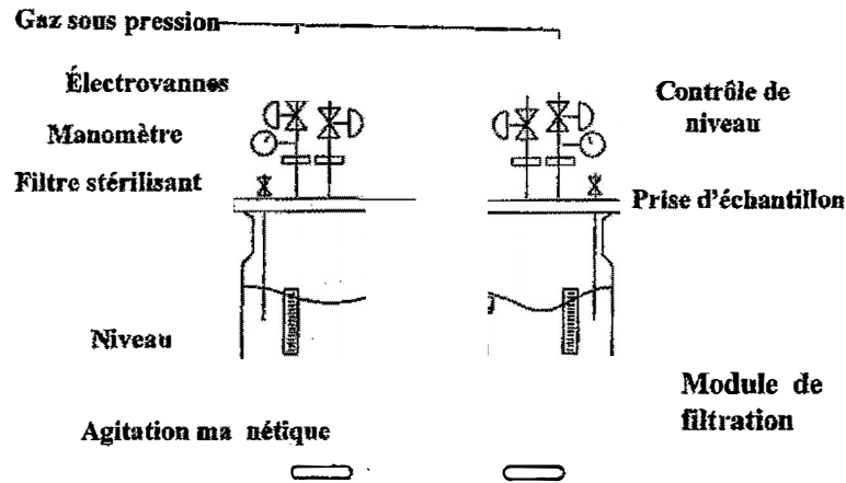
Figure 1 Schéma du bioréacteur Bioreactor design
