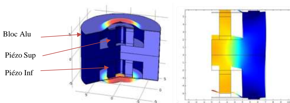
Figure 52 Simulations par éléments finis COMSOL du bloc piézo rapide [24]
