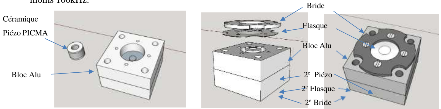
Figure 51 Bloc aluminium avec un des 2 piézos Vue en coupe de l'intégration des piézos dans le bloc aluminium avec les 2 flasques et les 2 brides Vue de l'ensemble « bloc piézo rapide » assemblé
