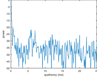
CP Cepstrum
