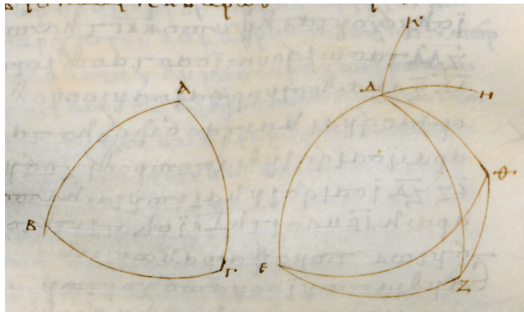
Pl. I. The diagram of Sph. I.13 in Theon, in Alm. VI.11. Firenze, Biblioteca Medicea Laurenziana, Ms. Plut. 28.18, f. 250v. Su concessione del MiBACT. È vietata ogni ulteriore riproduzione con qualsiasi mezzo.
