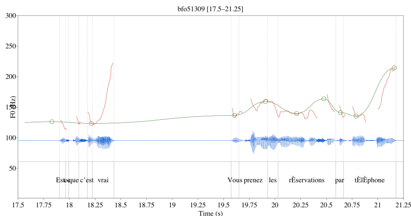
Figure 8: Old version of the automatic Momel algorithm for the utterance “Est-ce que c’est vrai ? Vous prenez les réservations par téléphone ?”. Raw (red) and modeled f_0 (green).
