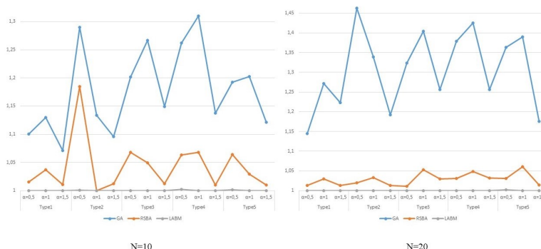
FIG. 1 – Variation des rapports d'approximation expérimentaux des différentes méthodes GA, RSBA et Algo : (i) à gauche de la figure pour n = 10 et, (ii) à droite de la figure pour n = 20 .
