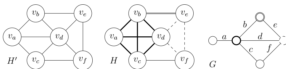
FIG. 1 – Le graphe H' à gauche n'est pas un linegraph, mais est à une distance d'édition 1 d'un linegraph, par exemple H qui est le linegraph de G . Les décorations des arêtes de H et des nœuds de G sont une couverture en clique de H , introduite dans la section 3.
