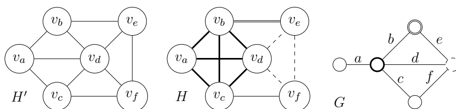
FIG. 1 – Le graphe H' à gauche n'est pas un linegraph, mais est à une distance d'édition 1 d'un linegraph, par exemple H qui est le linegraph de G . Les décorations des arêtes de H et des nœuds de G sont une couverture en clique de H , introduite dans la section 3.
