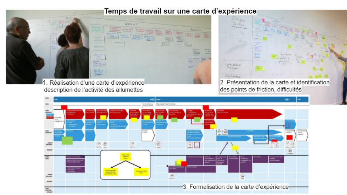
Figure 2. La carte d'expérience utilisée dans le projet PREMaTT
