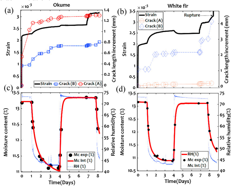
Fig. 5. Strain test 2 (a) Okume; (b) White fir; (c) Okume; (d) White fir.
