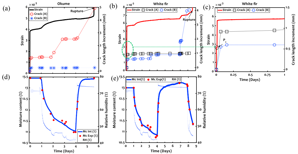
Fig. 4. Strain test 1(a) Okume; (b) White fir; (c) Okume; (d) White fir (e) Zoom White fir.
