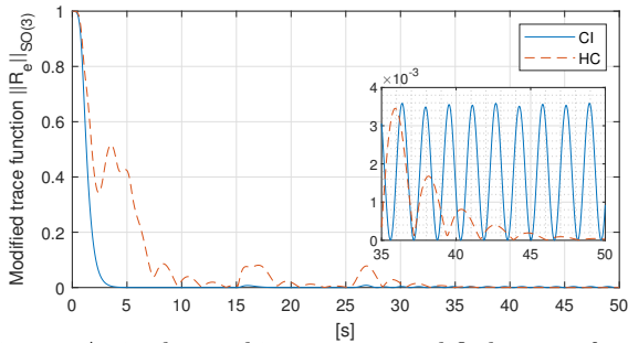
Fig. 3. Attitude tracking error: modified trace function ( \|R_e\|_{SO(3)} ).
