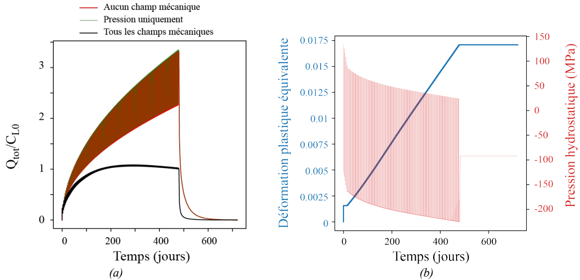
Figure 4. (a) Évolution de la quantité totale d'hydrogène Q_{tot} = \int (C_L + C_T)dV normalisée par C_{L,0} en fonction du temps, pour les trois configurations, (b) déformation plastique équivalente (bleu) & pression hydrostatique (rouge) sur le point A (voir la Figure 1c) au cours du temps dans le cas où tous les champs mécaniques sont résolus.
