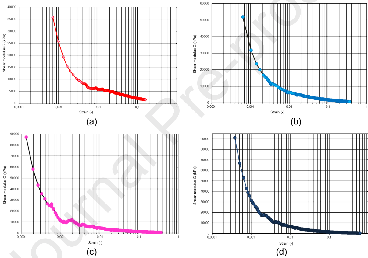
Fig. 21. Shear Modulus Degradation. (a) Test 1, (b) Test 2, (c) Test 3 et (d) Test 4
