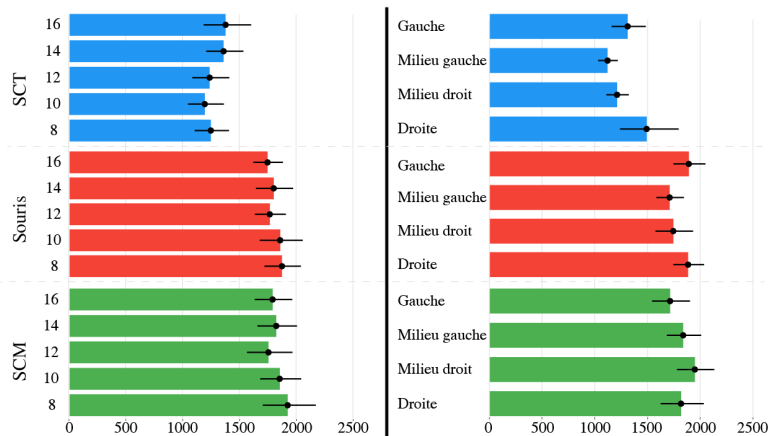
Figure 5: Affinement par technique, en fonction du nombre d'éléments (Gauche) et de la position de la cible (Droite). Toutes les barres représentent des IC à 95 %.
