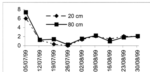
Fig. 6 : Variations des quantités relatives (%) du \alpha -pinène en milieu fermé.
