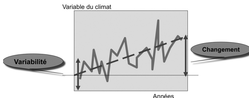
Augmentation de la variabilité climatique et de la fréquence des événements extrêmes
