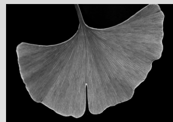
Le Ginkgo Biloba, un des premiers gymnospermes, a des propriétés antioxydantes : il est utilisé comme anti vieillissement et favorise la circulation veineuse. Il a aussi des propriétés anticancéreuses recherchés par les laboratoires pharmaceutiques, notamment pour la lutte contre le cancer du sein.
