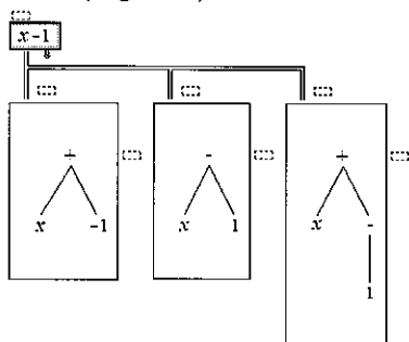
Figure 7. Multiplicité d'arbres représentant une même expression algébrique.
