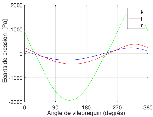
Figure 8 : Ecart de pression dans les échangeurs pour des températures de source et puits de 473 K et 288 K
