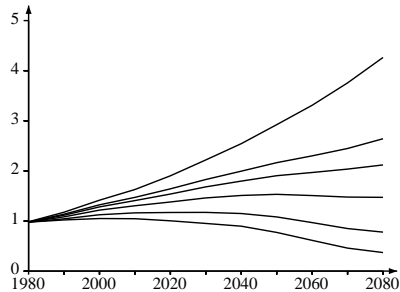
25.4. ábra. Demográfiai előrejelzések (milliárdokban) az egy nőre jutó gyermekek átlagos számára vonatkozó különböző hipotézisek alapján. Alulról felfelé: b = 1,0; 1,5; 2,0; 2,3; 2,5; 3,0 .
