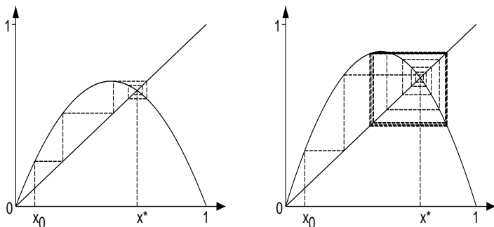
24.3. ábra. Az y = f(x) = rx(1-x) függvény, az y = x egyenes, az x^* egyensúlyi helyzet és az x_{n+1} = f(x_n) által meghatározott sorozat. Balra: r = 2,75 , a sorozat x^* -hoz tart. Jobbra: r = 3,4 , az egyensúlyi helyzet x^* instabil, és a sorozat egy 2 periódusú ciklushoz tart.
