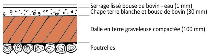
Différentes couches d'une terrasse de takienta
