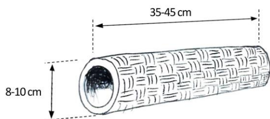
Dimensions courantes d'une gargouille
