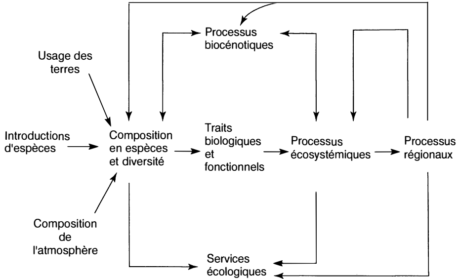
Figure 2. — La dynamique des systèmes écologiques est soumise à l'action des hommes (à gauche). Ce schéma souligne les liens, importants et mal connus, entre les espèces et les processus écosystémiques (production, décomposition, cycles de la matière). Les processus biocénétiques incluent la prédation, la compétition, le parasitisme, le mutualisme. Quant aux services écologiques, ils représentent les bénéfices que l'homme tire gratuitement du fonctionnement des écosystèmes (régulation des climats, fertilité des sols, pollinisation, recyclage des éléments...). D'après Chapin et al. , 1997.
