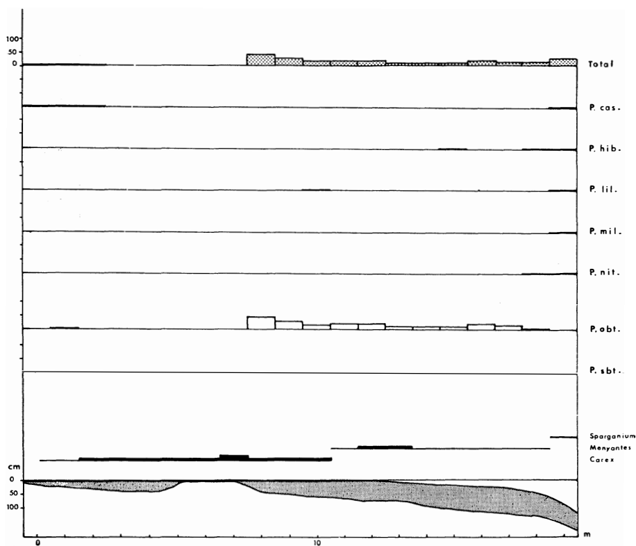
Fig. 9. — Transect G.
