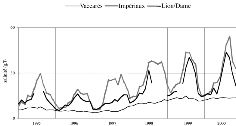
Figure 3. — Evolution de la salinité des étangs du système Vaccarès de 1995 à 2000
