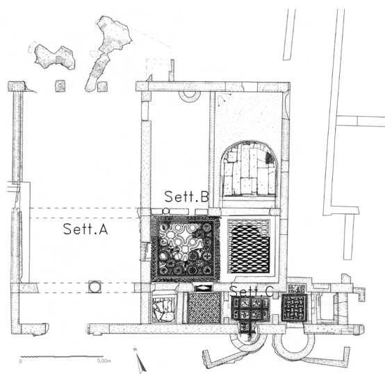
Fig. 13. Balneum di Musiciolus (pianta: Marcello Turci, scala 1:50 con sovrapposizione dei mosaici pvmimentali tratti da Ostia [Parco Archeologico di Ostia Antica - PA-OANT, Archivio Disegni, plan. n. 13942 (autore A. Pascolini)])
