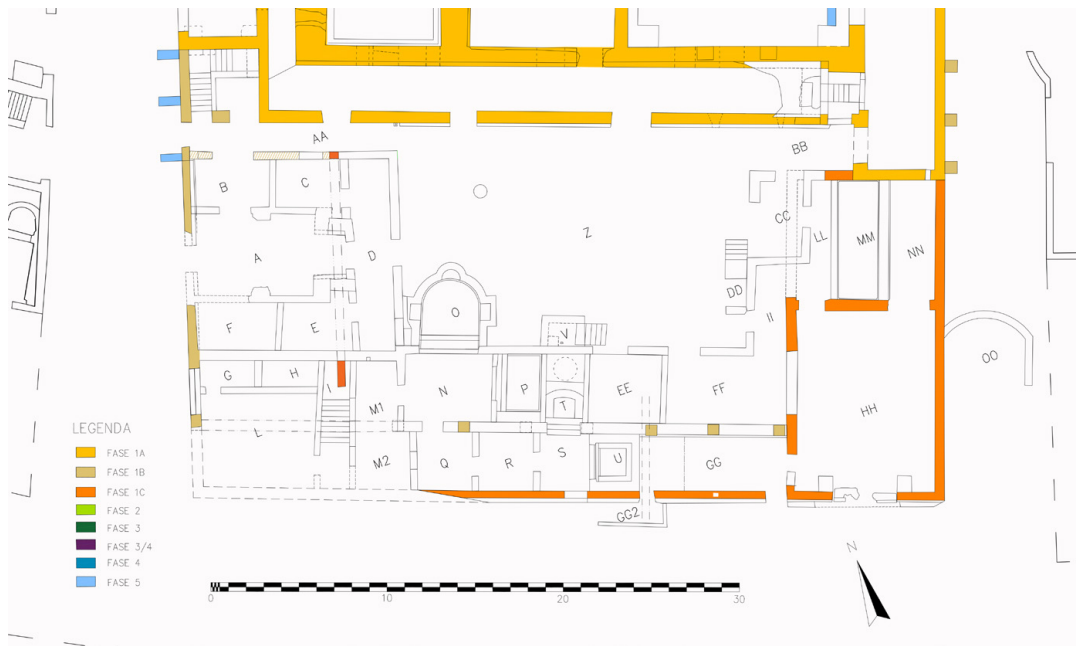
Fig. 3. Edificio IV X, 2: fase 1, et  antonina (  Marcello Turci)
