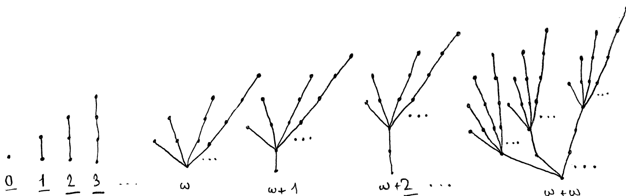
FIGURE 1 – Arbres ordinaux.
