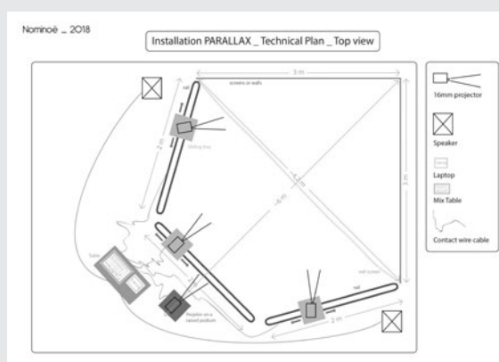
Plan d'installation technique de Parallax (vue de dessus), Nominoë, 2018
