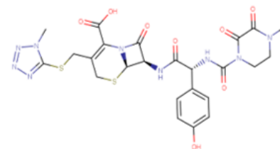
Cefoperazone (CFZ)
