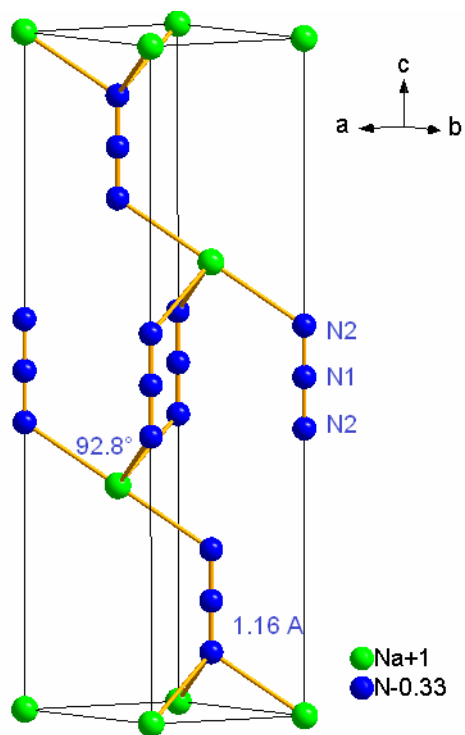
a) rh -NaN 3
