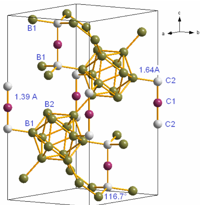
b) h -B 36 C 9
