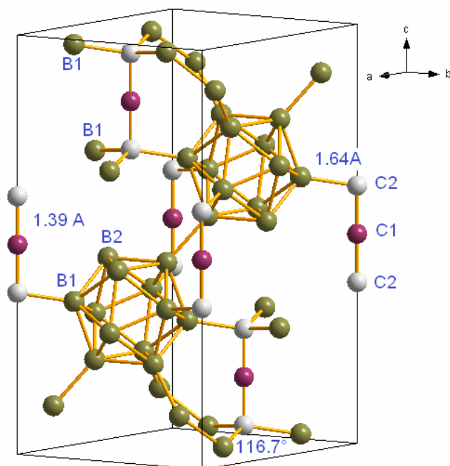
b) h\text{-B}_{36}\text{C}_9
