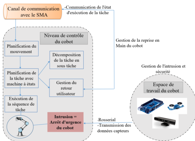
Figure 5. Interaction et exécution du service au niveau exécutif du système
