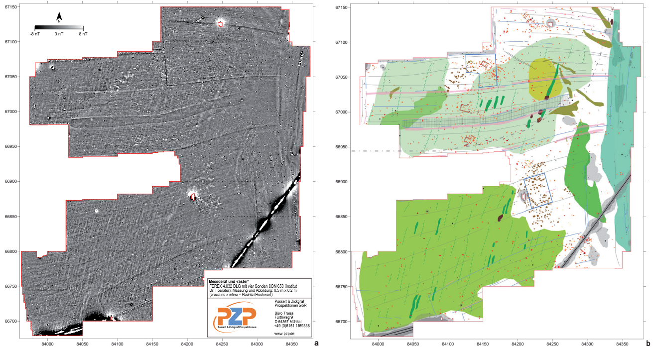
Fig. 3 - Représentation de la prospection géophysique en niveaux de gris (a) et interprétation (b) en anomalies géologiques ou pédologiques (couleurs froides) et en structures archéologiques (couleurs chaudes), dont le signal varie en intensité selon les réglages du magnétomètre. En bleu, les deux zones sélectionnées pour cette campagne de fouille. Fond de carte et analyses des résultats : B. Zickgraf et B. Schroth (PZZ).
