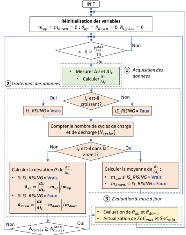
Fig. 8: Organigramme de l'algorithme pour l'indétermination des limites de SoC_{min} et SoC_{max} qui garantissent l'opération dans la zone linéaire.
