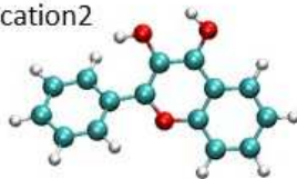
3HF cation2
