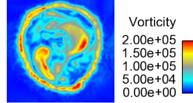
(b) Vorticity
