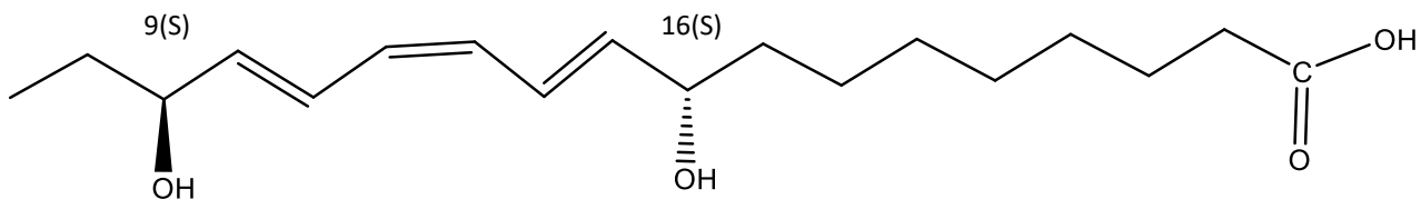
9(S),16(S)-diOH-10 E ,12 Z ,14 E -18:3
