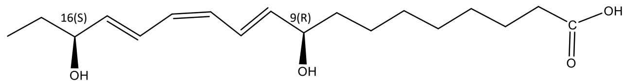
9(R),16(S)-diOH-10 E ,12 Z ,14 E -18:3
