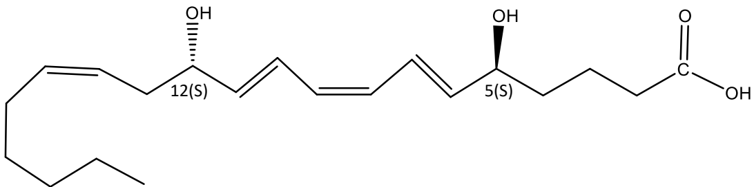
5(S),12(S)-diOH-6 E ,8 Z ,10 E ,14 Z -20:4 (LTBX)
