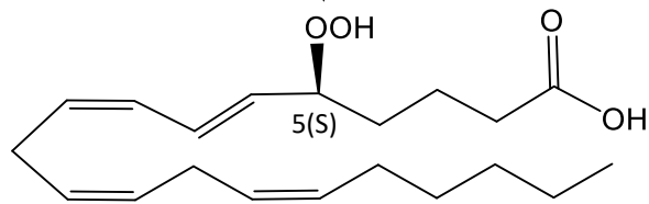
5(S)-OOH-6E,8Z,11Z,14Z-20:4 (5-HpETE)
