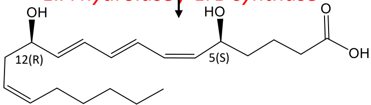
5(S),12(R)-diOH,6Z,8E,10E,14Z-20:4 (LTB4)
