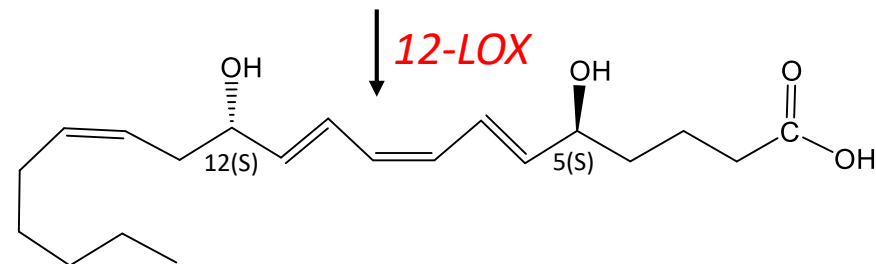
5(S),12(S)-diOH-6E,8Z,10E,14Z-20:4 (LTBX)
