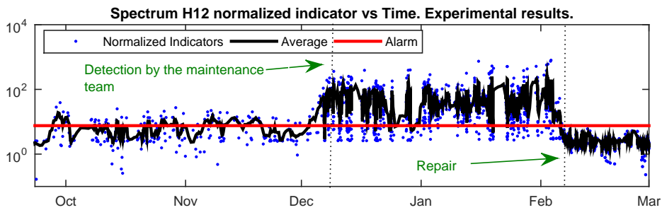
(d) IAS H12 Normalized indicator. Experimental results.
