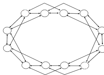
FIG 1. Réseau de 12 nœuds en topologie i+1, i+2
