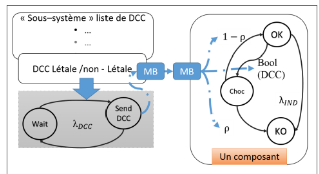
FIG 3. Modélisation des DCC avec PyCATSHOO
