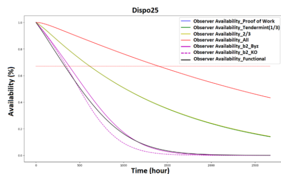
FIG.7 Evolution des disponibilités moyennes en fonction du temps selon les 7 observateurs
