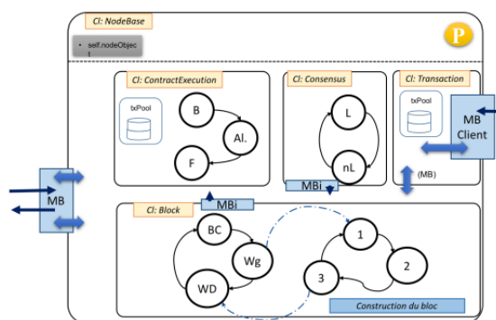
FIG 2. Modélisation fonctionnelle avec PyCATSHOO
