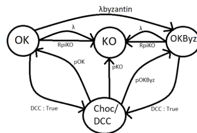
FIG.4. Automate « aBasicByzantineComponent » avec Défaillances byzantines
