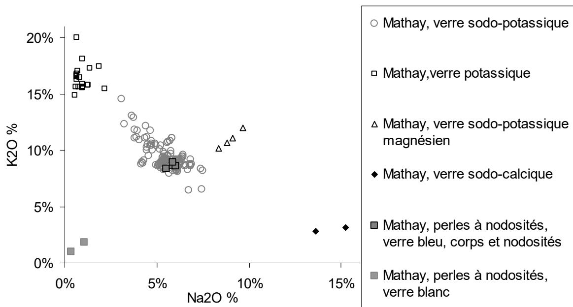
Figure 2 : diagramme Na 2 O vs K 2 O pour les perles de Mathay. La présence de quatre types de verres bleus est observée à Mathay.
