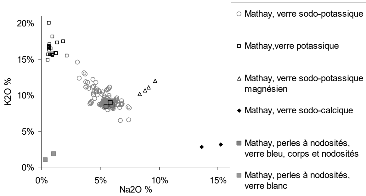
Figure 2 : diagramme \text{Na}_2\text{O} vs \text{K}_2\text{O} pour les perles de Mathay. La présence de quatre types de verres bleus est observée à Mathay.
