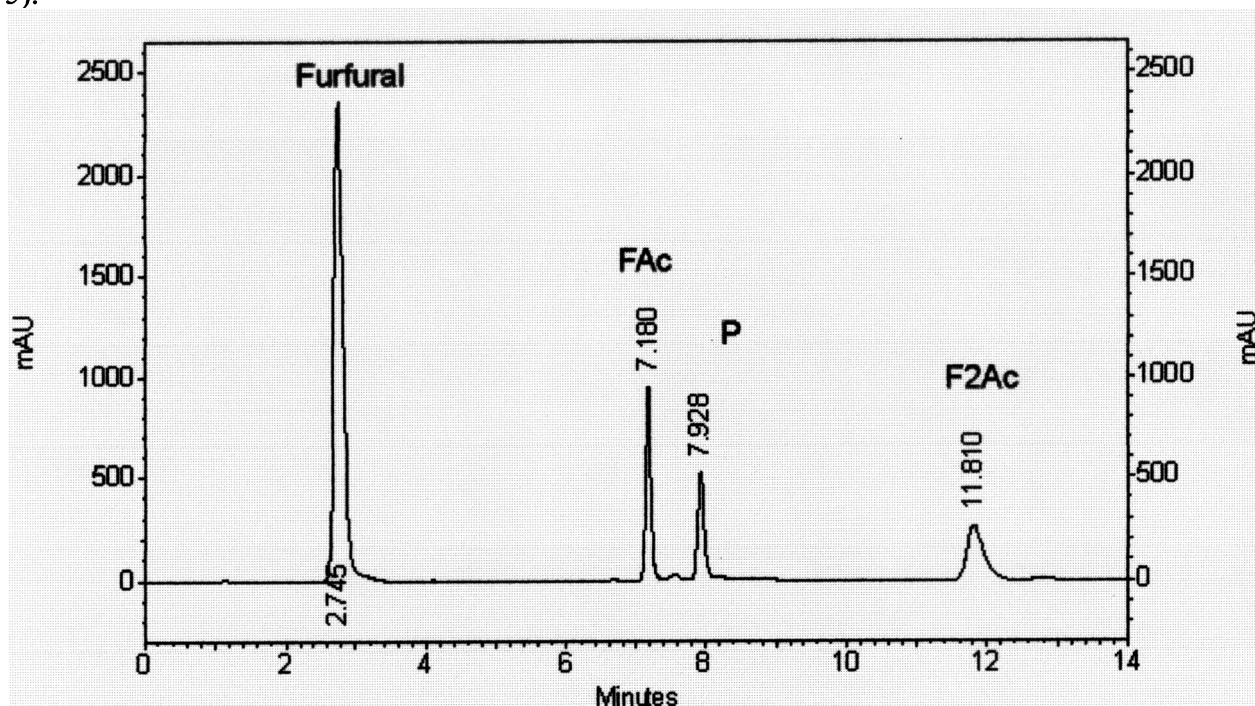
Figure 5 : Chromatogramme CLHP obtenu pour un prélèvement à 10 min d'une réaction à 34°C
