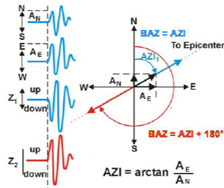
Image 3. Cette figure est issue de la publication (doi: 10.2312/GFZ.NMSOP-2_IS_11.1) de Jens Havskov (Université de Bergen), Peter Bormann (German Research Centre for Geosciences), et Johannes Schweitzer (NORSAR). Elle décrit la détermination de l'azimut et du back-azimut à partir d'un exemple simplifié de l'enregistrement de l'onde P sur trois composantes d'un même capteur.
