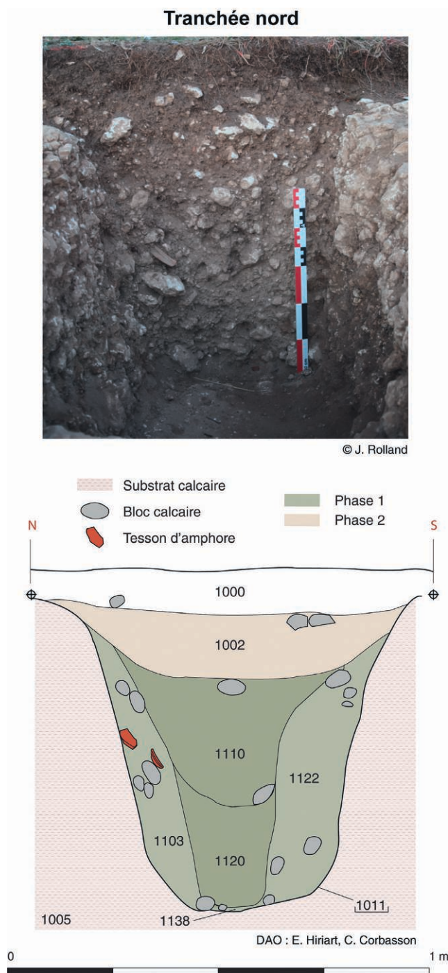
Figure 7 : Coupe à travers la tranchée nord de l'enclos F6 (cliché : J. Rolland, DAO : C. Corbasson, E. Hiriart).
