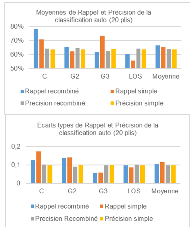
Fig. 8. métriques d'entraînement de la BDD 2k avec 20 plis avec métadonnée complexe et simple.
